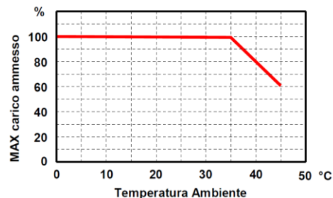
Fig. 1 - Declassamento del carico massimo ammesso in funzione della temperatura ambiente:
